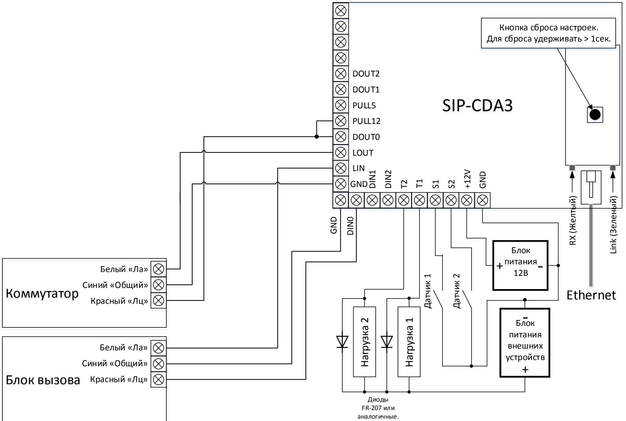
Схема подключения SIP-CDA3 к домофонам Факториал.
